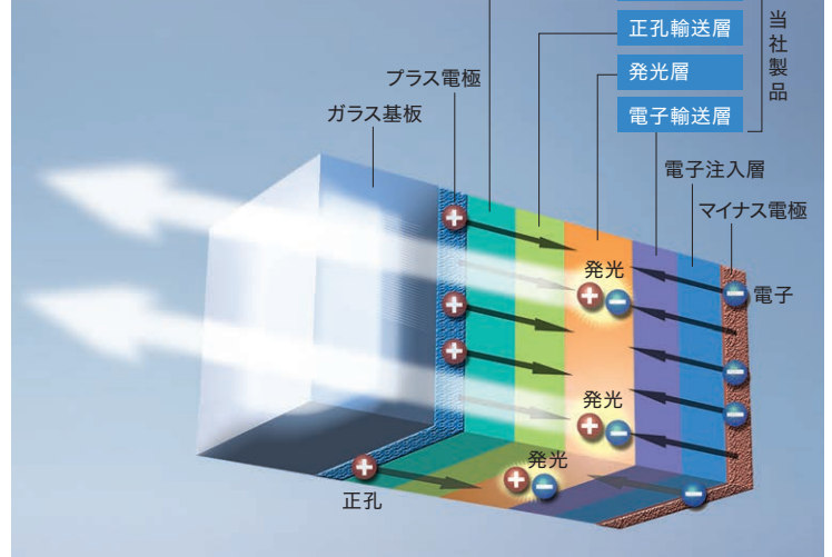
有機デバイスの構造
