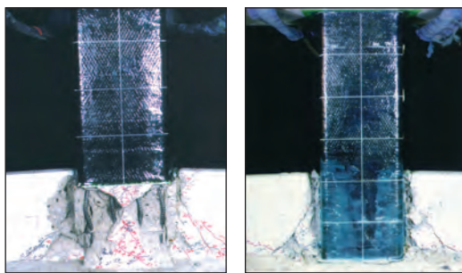
補強なし
